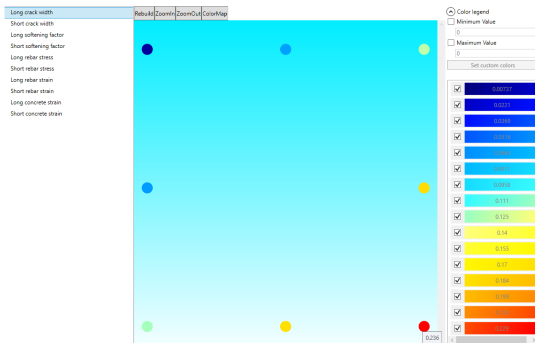
Рисунок 14-30. Результаты расчета на раскрытие трещин в виде изополей.
