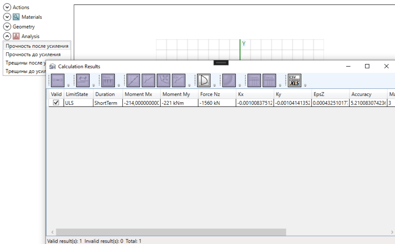
Рисунок 14-24. Результаты расчета прочности после усиления.
