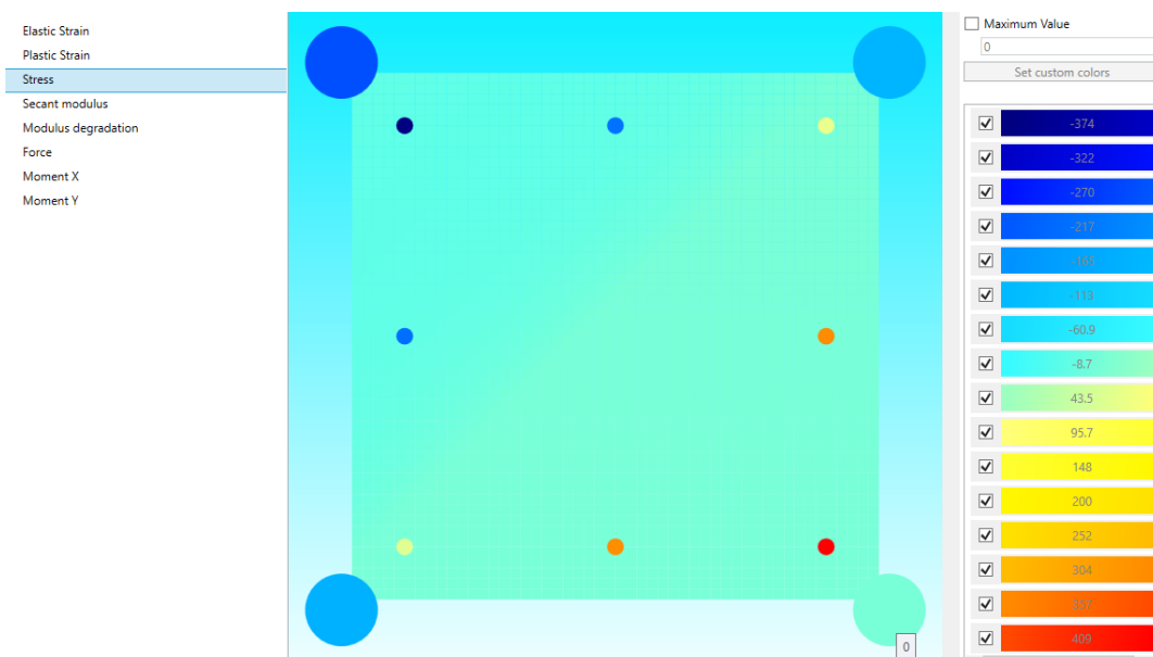
Рисунок 14-28. Изополя напряжений в элементе при нагрузке, близкой к предельной.
