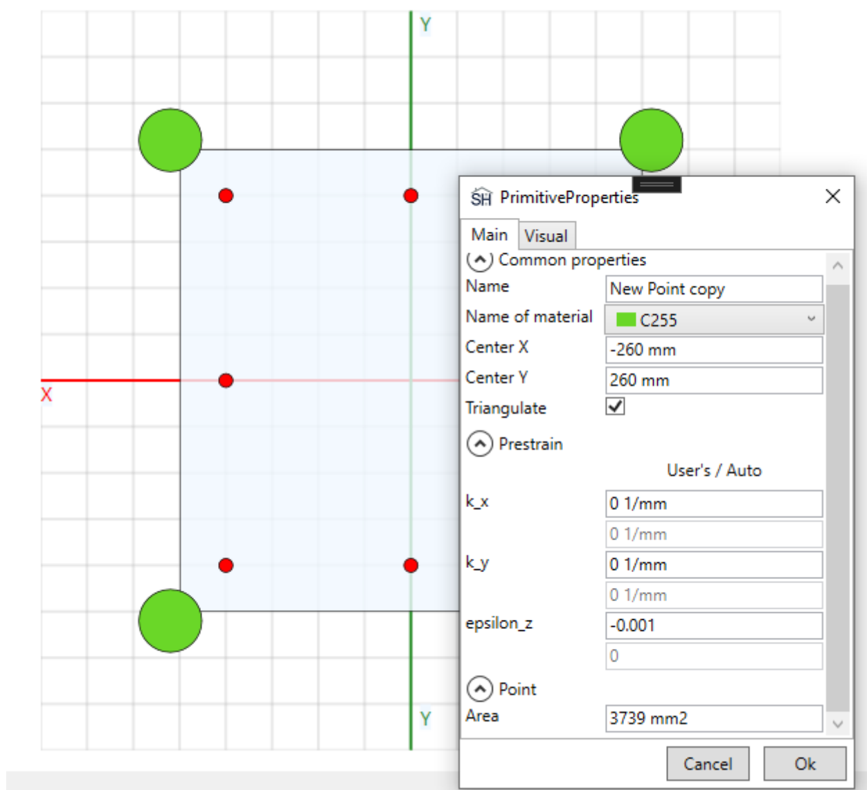
Рисунок 14-22. Свойства примитивов, соответствующих стальным уголкам усиления.
