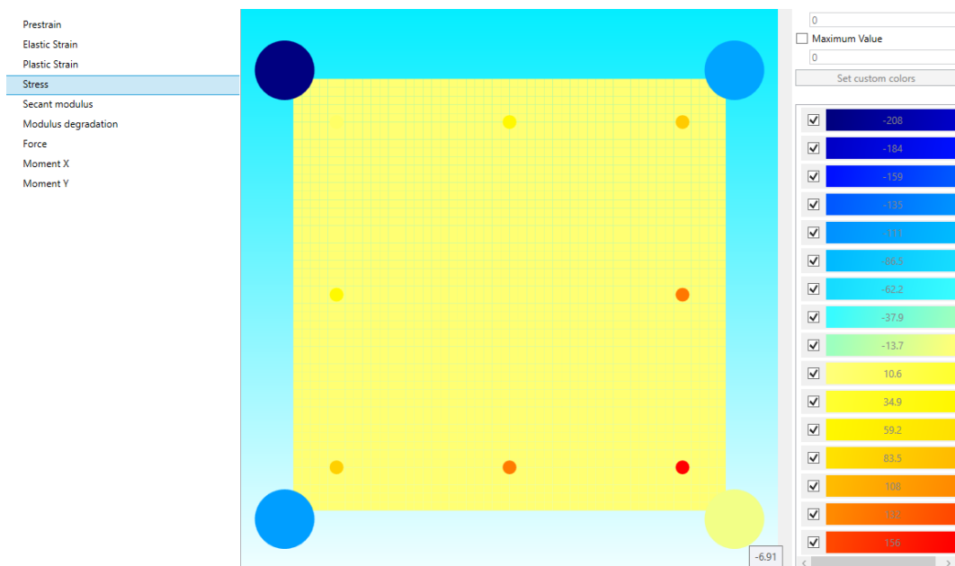
Рисунок 14-27. Изополя напряжений в элементе при заданной нагрузке.
